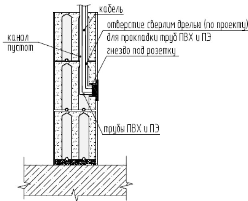
б) Горизонтальное сечение.
